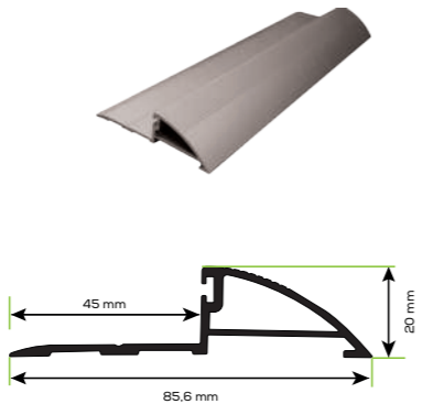
OPTION SEUIL ALU
