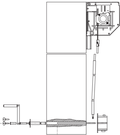
OPTION MANOEUVRE DE SECOURS EXTÉRIEURE - INTÉRIEURE
