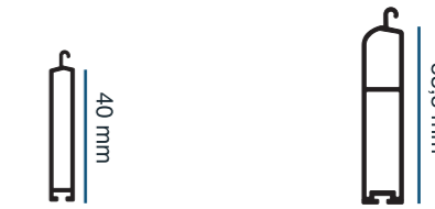
Petite lame finale pour tablier RS 41 SW - PVC 40 Bio Grande lame finale pour tablier RS 52
