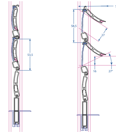
Volet semi-ouvert
