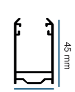
27 mm Z14 pour tablier lames : RS 52 - PVC 52
