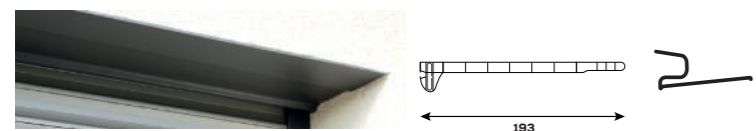
Sous-face Cache-rail PVC
