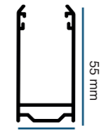
27,5 mm Z55 à partir de 3500 mm RS 52 sur demande
